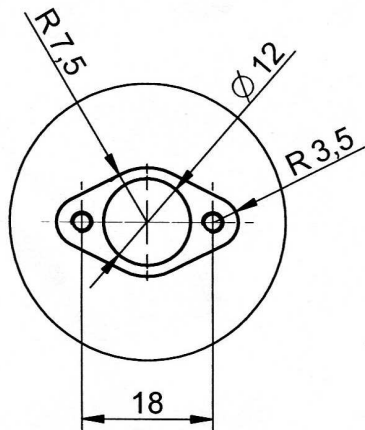
Detalj A 1:1
